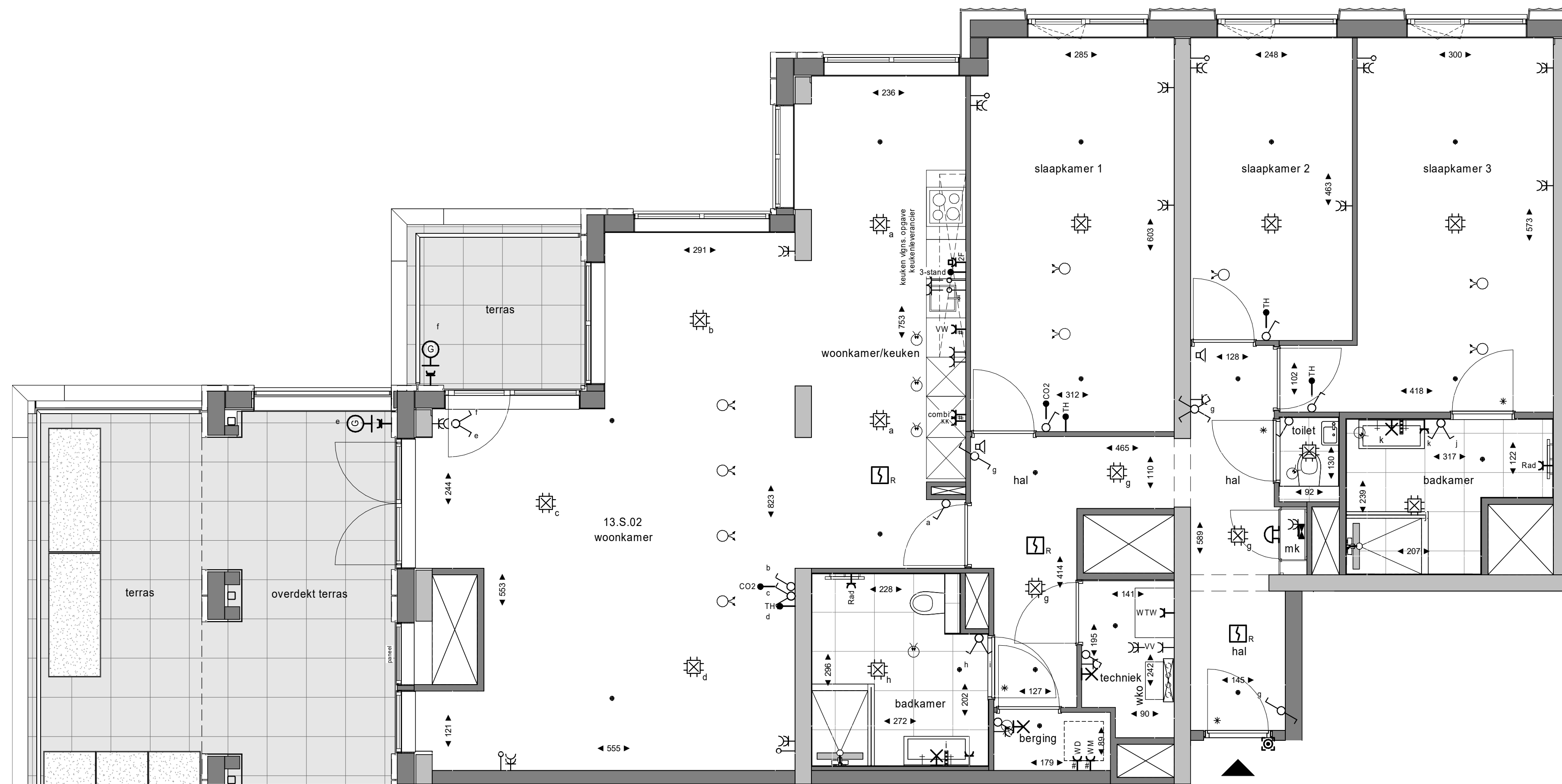
plattegrond 1 : 50 13e verdieping
